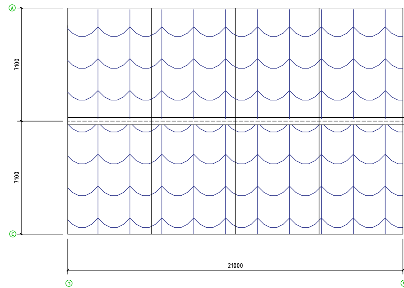
屋面彩钢瓦铺设平面示意图 1:100
