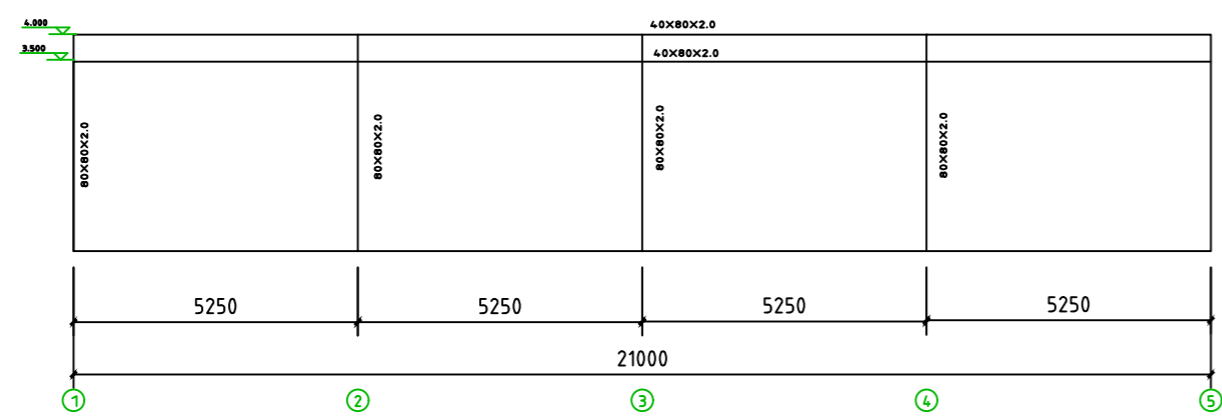
立面示意图2 1:100
