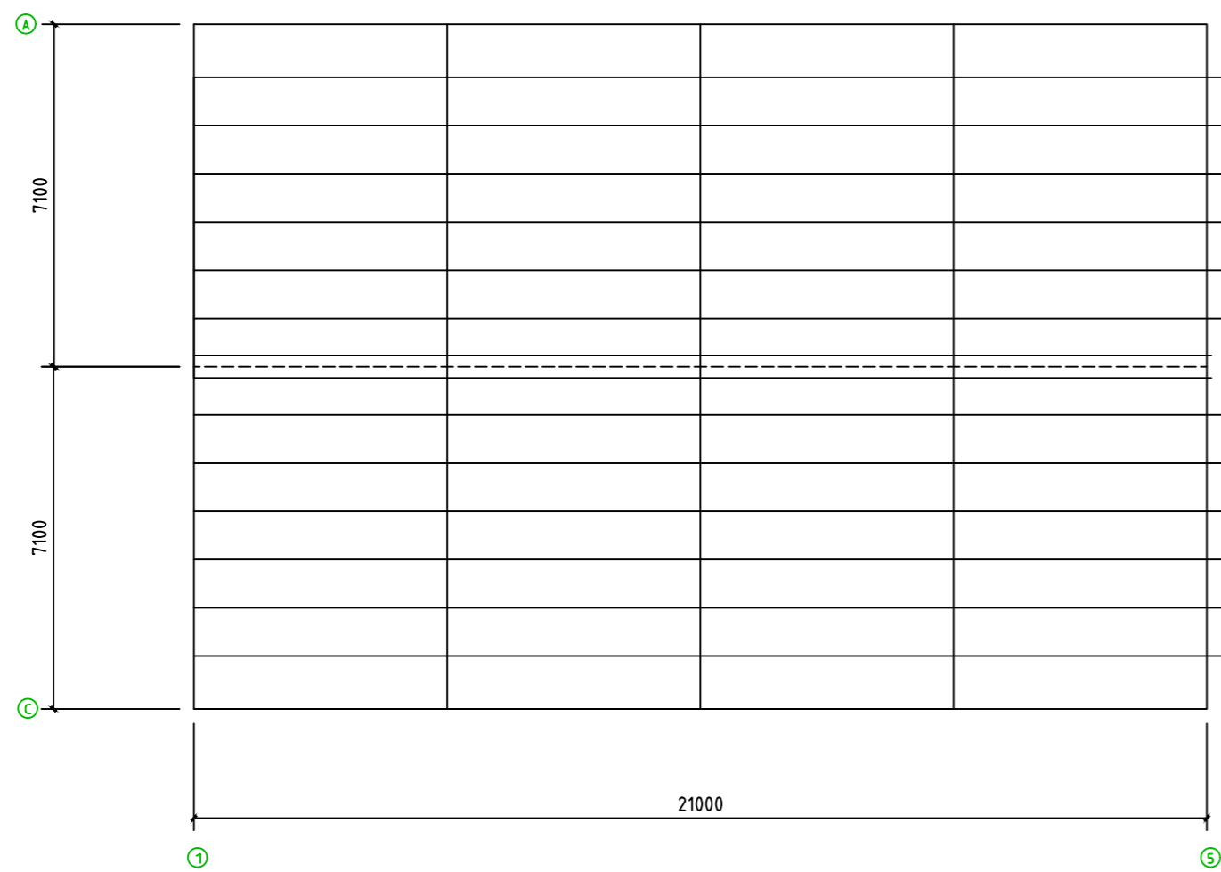
屋面骨架平面示意图 1:100
